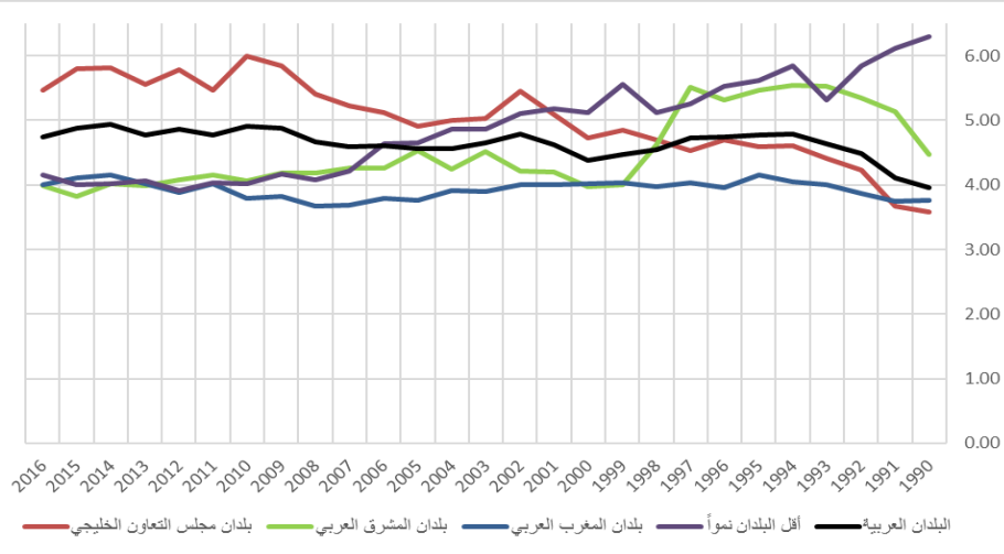
حصة الطاقة المتجددة من مجموع الاستهلاك النهائي للطاقة في المنطقة العربية وفقاً لمجموعات البلدان (بالنسبة المئوية)
