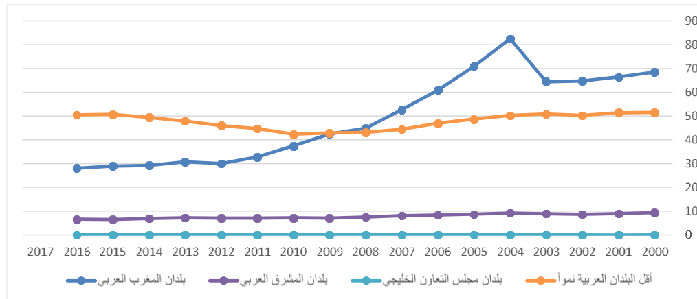
حصة الطاقة المتجددة من مجموع الاستهلاك النهائي للطاقة في المنطقة العربية وفقاً لمجموعات البلدان (بالنسبة المئوية)
