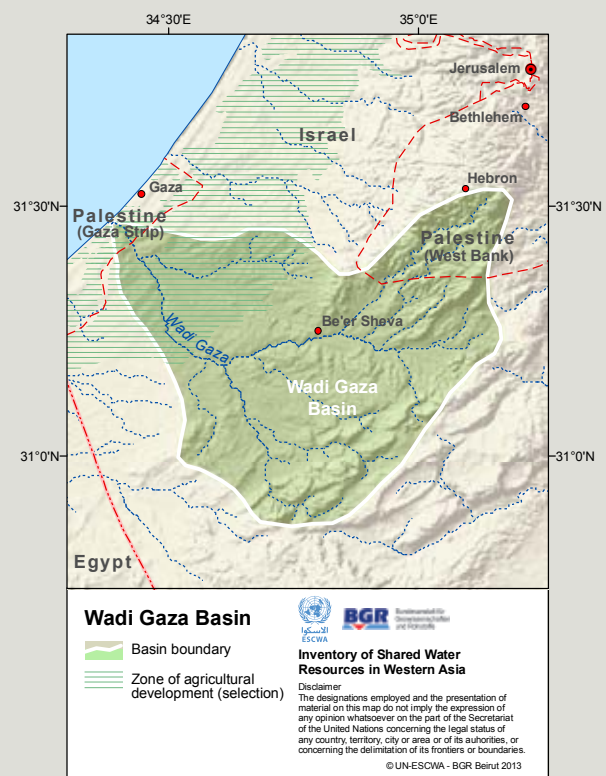
Figure 2. Wadi Gaza Basin
