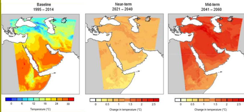
متوسط التغير في درجة الحرارة السنوية مقارنة بفترة خط الأساس
